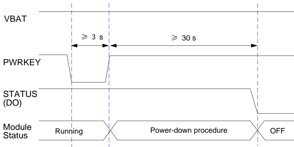
图 14：关机时序图
