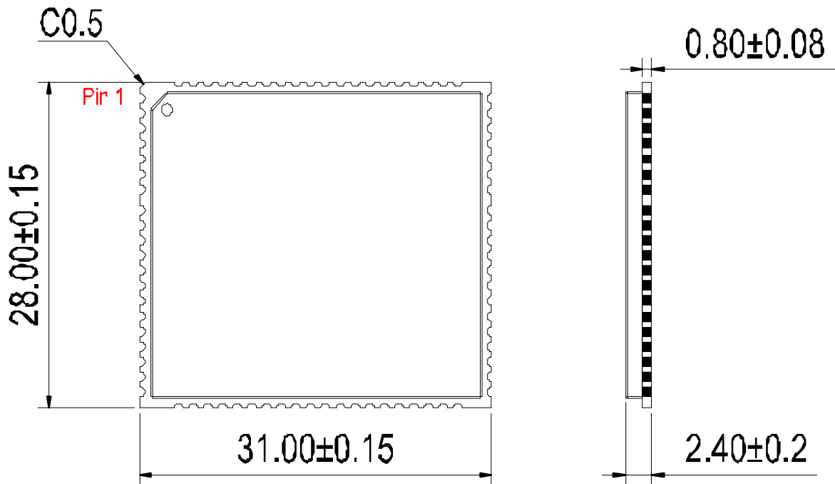
图 39：模块俯视及侧视尺寸图
