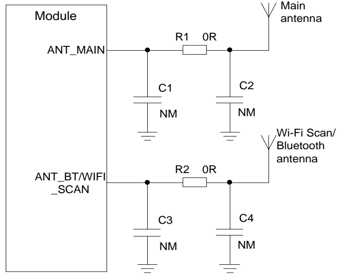
图 30: 射频参考电路
