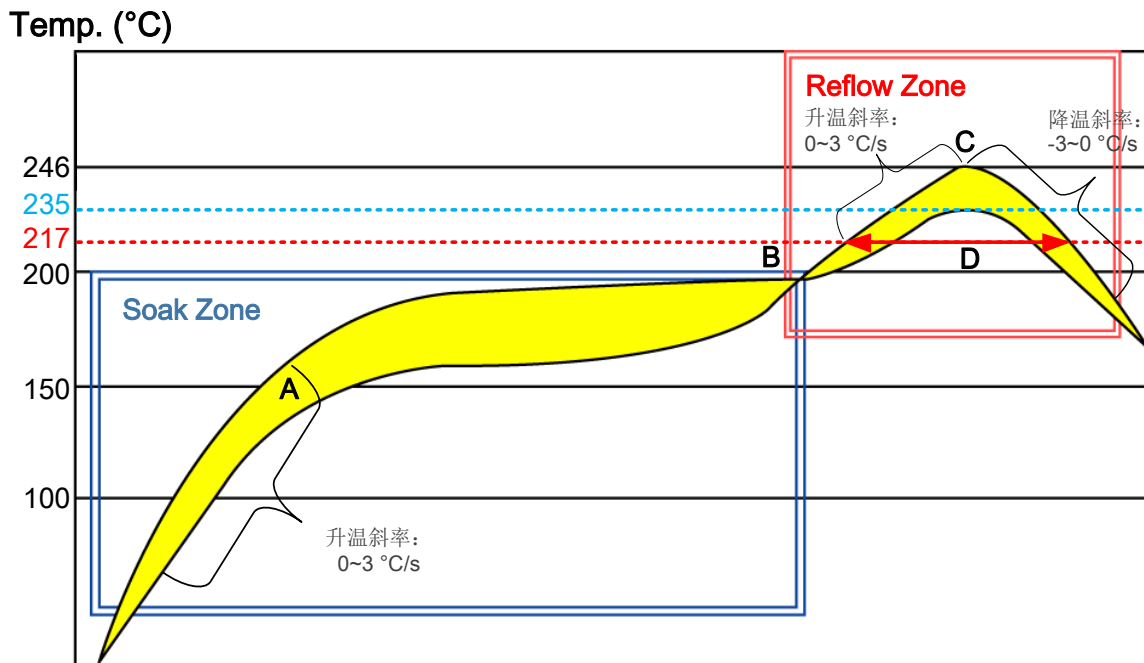
图 43：回流焊温度曲线
