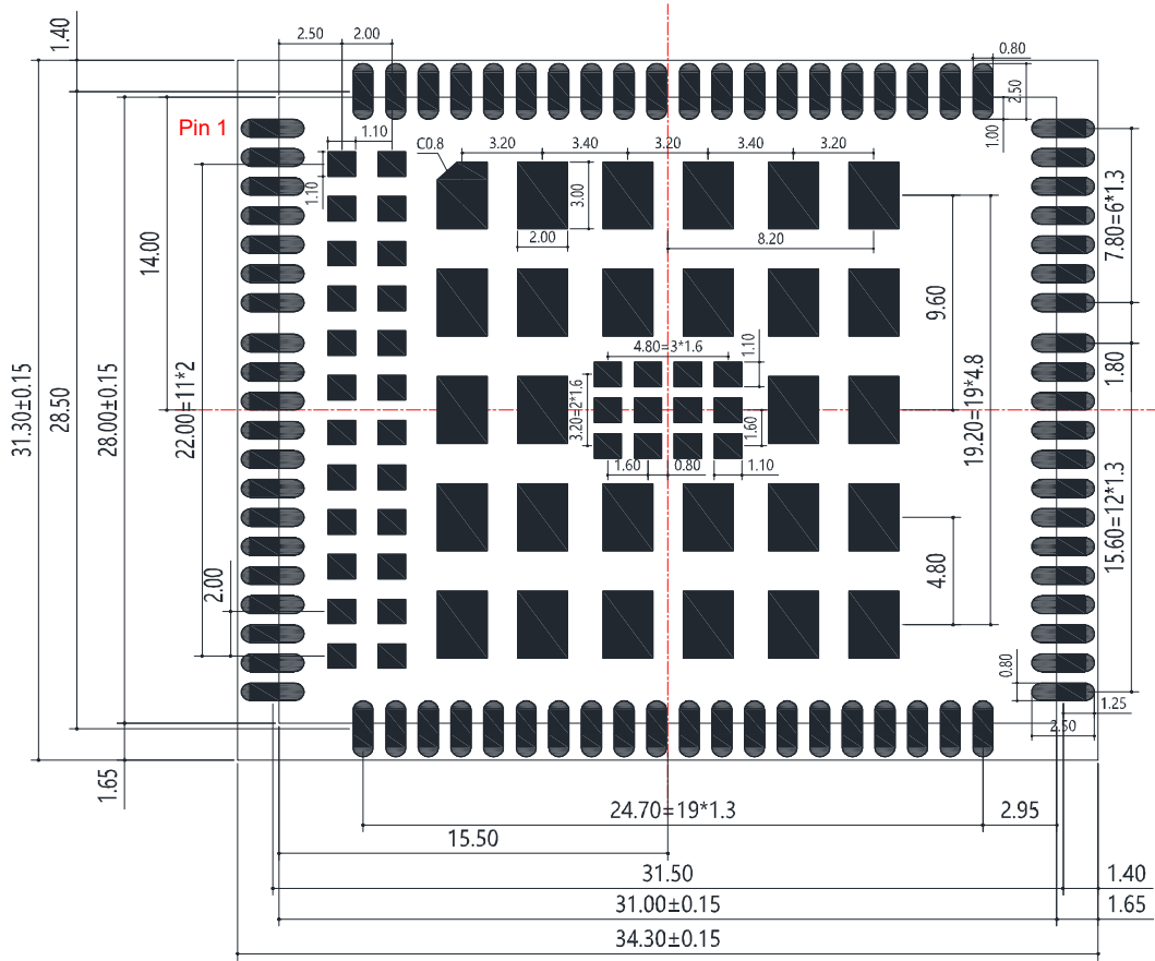
图 41：推荐封装（俯视图）
