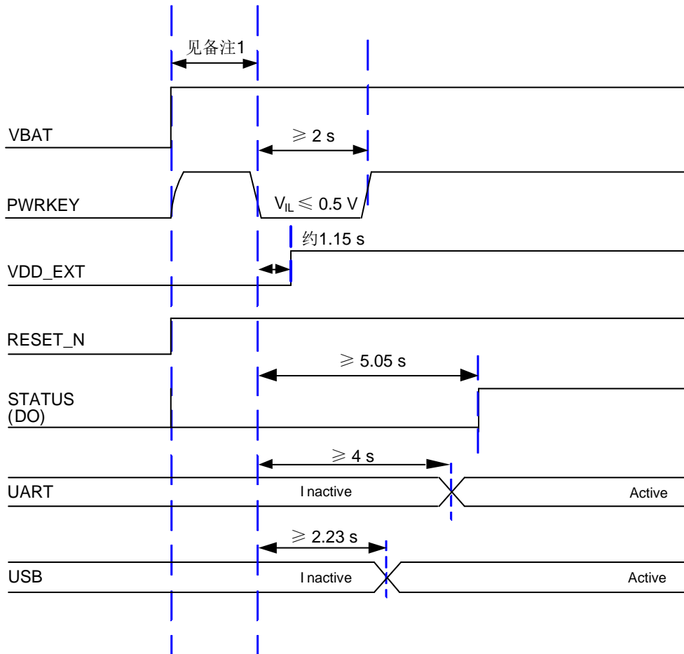
图 13: 开机时序图
