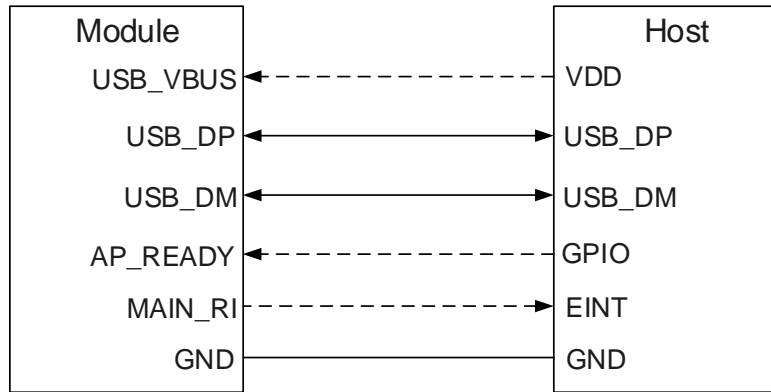
图 6：带 MAIN_RI 功能的睡眠应用
