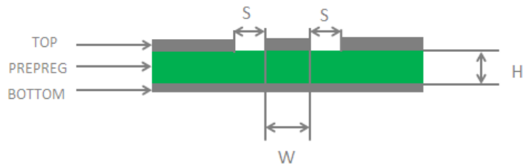
图 33: 两层 PCB 板共面波导结构
