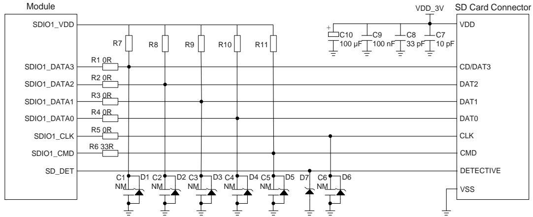
图 26: SD 卡接口电路参考设计
