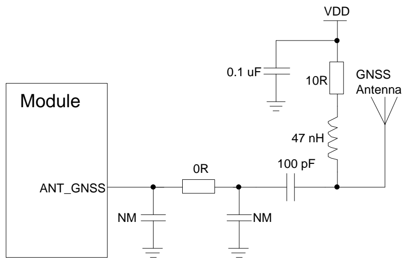
图 31: GNSS 天线参考电路
