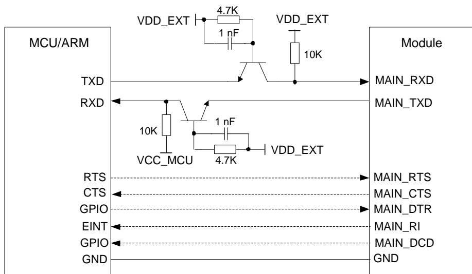
图 22：三极管电平转换参考电路
