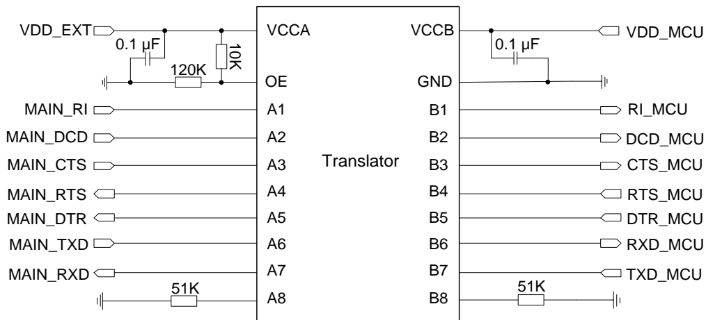
图 21：电平转换芯片参考电路
