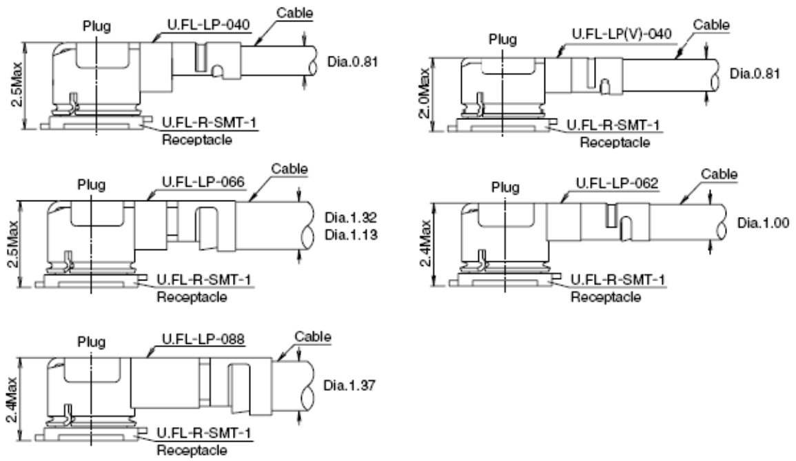
图 38：射频连接器安装图（单位：毫米）
