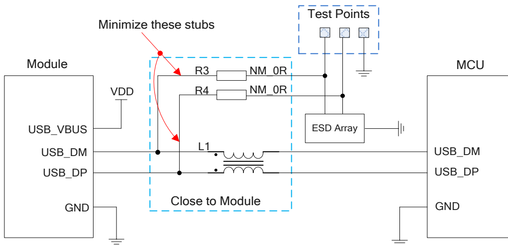
图 20: USB 接口参考设计
