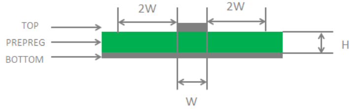
图 32: 两层 PCB 板微带线结构
