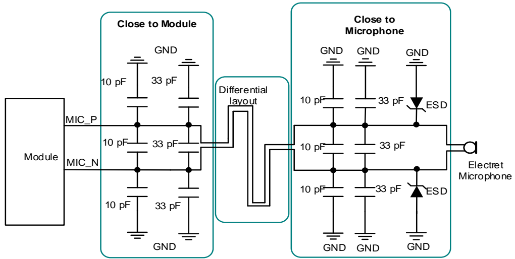
图 24: 麦克风接口参考电路
