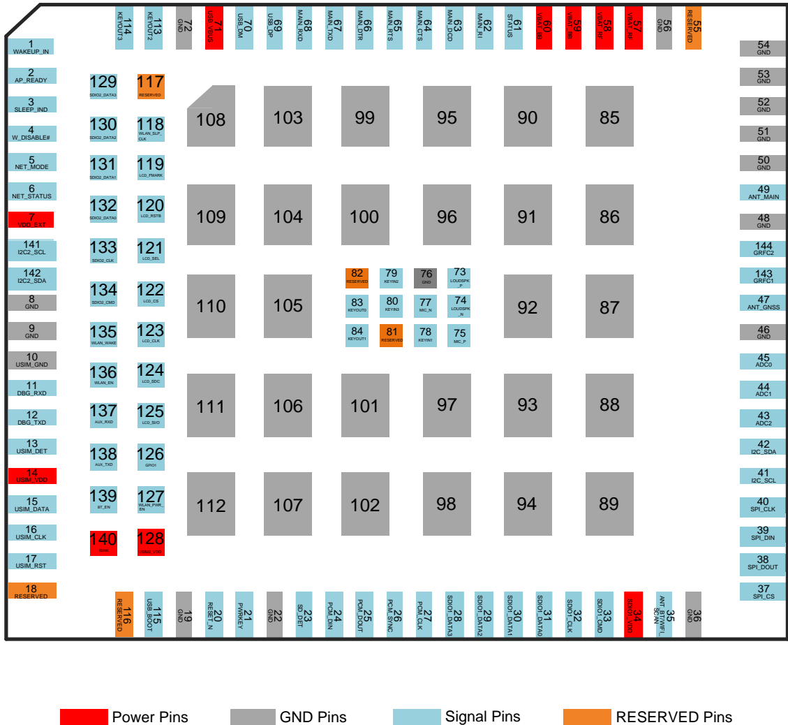
图 2: EC200U 系列模块引脚分配俯视图
