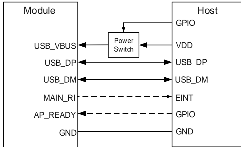
图 7：不支持 USB 挂起功能的睡眠应用
