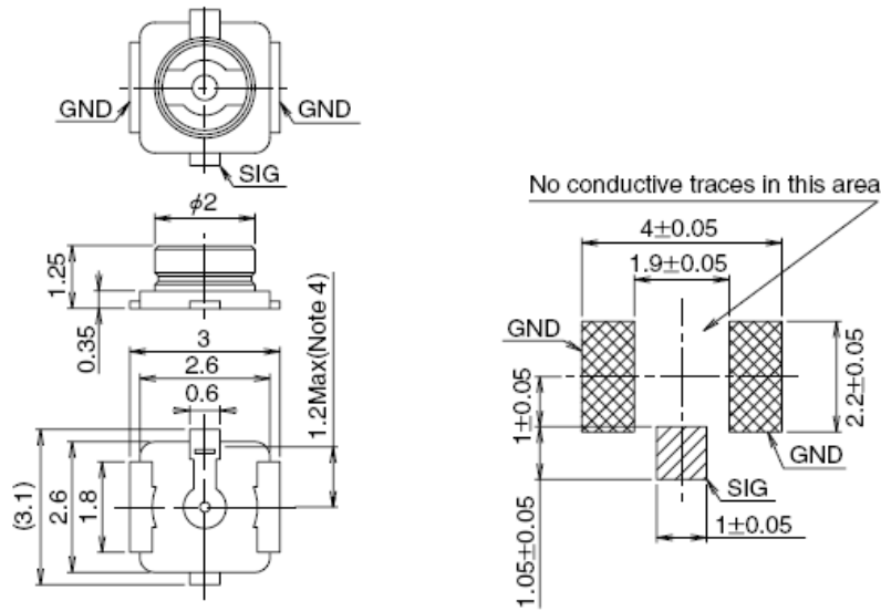
图 36: 天线座尺寸 (单位: 毫米)
